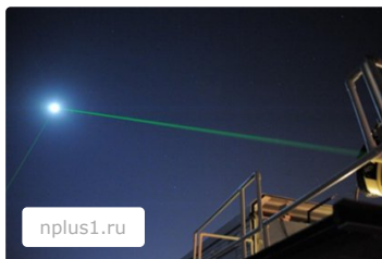
Лазерное зондирование Луны подтвердило фундаментальную симметрию теории относительности
